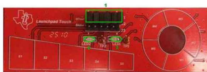
图 4. 触摸感应子卡设置示意图
